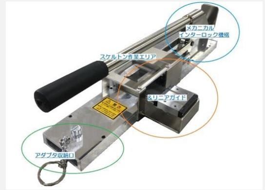
CPUをスムーズにセット・殻割・簡単排出（操作レバーを左右に振る）
