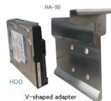
DB-60PRO NSA準拠のV&M (4点孔) HA-50アダプタを利用した破壊動作
