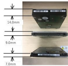
DB-80SSD及びDB-50SSD用新アダプタの仕様
